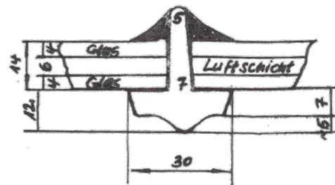
Innensteg
